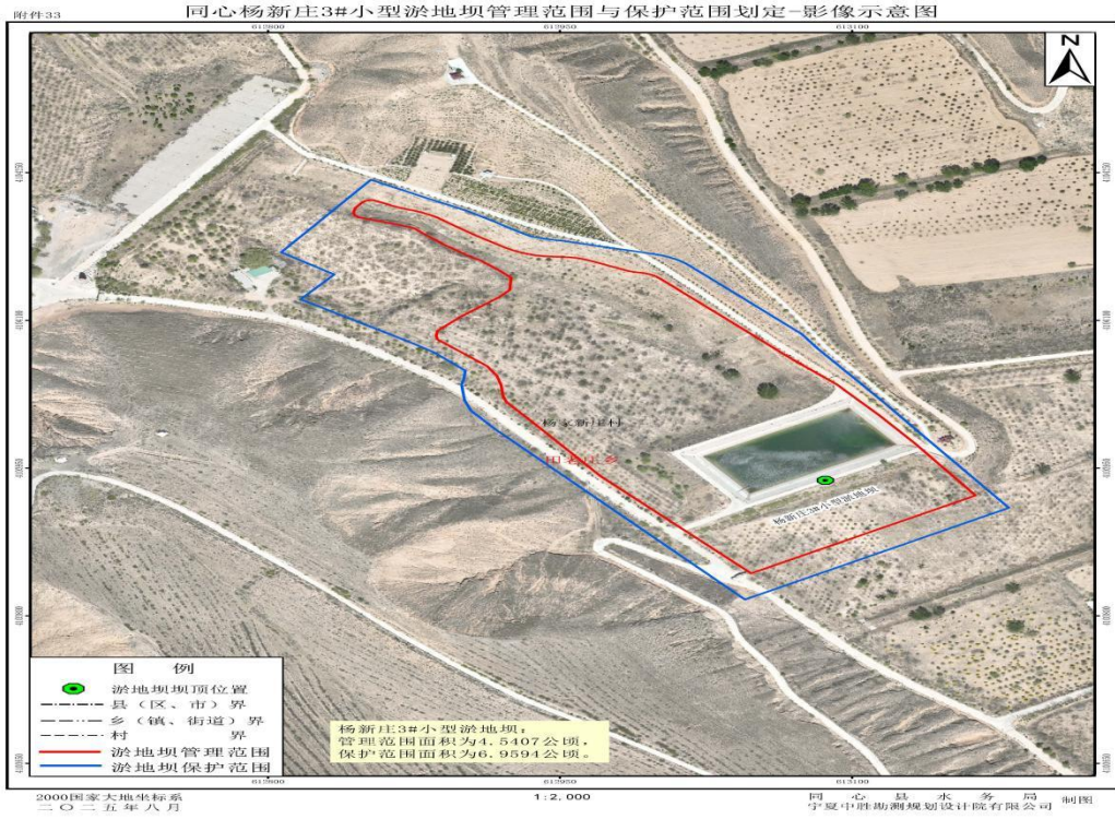
1-33 同心县杨新庄3#淤地坝管理与保护范围划定成果影像示意图
