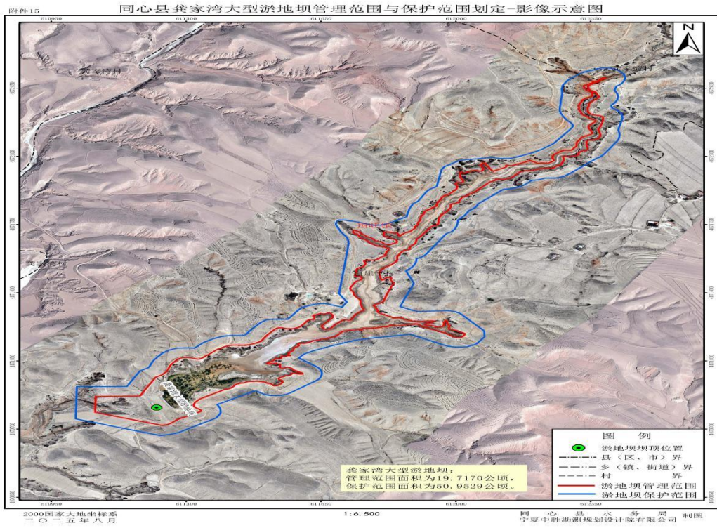
1-15 同心县龚家湾淤地坝管理与保护范围划定成果影像示意图
