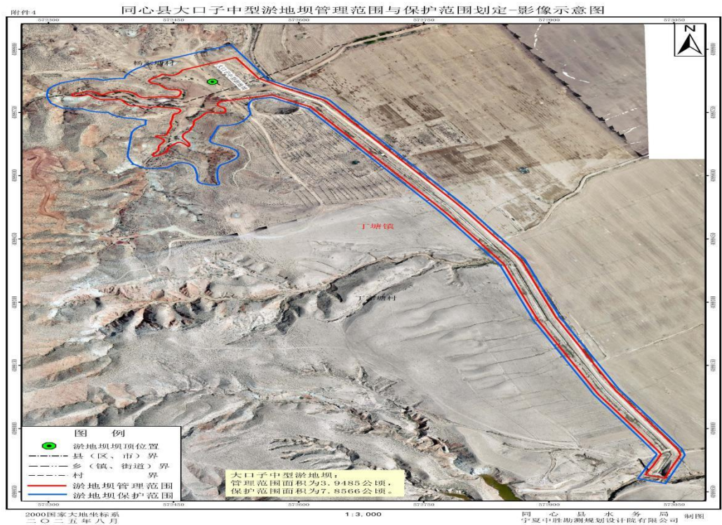
1-4 同心县大口子淤地坝管理与保护范围划定成果影像示意图
