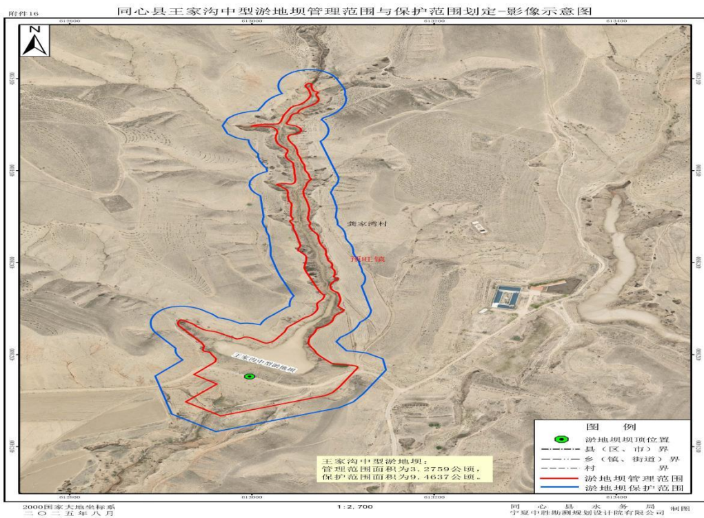
1-16 同心县王家沟淤地坝管理与保护范围划定成果影像示意图
