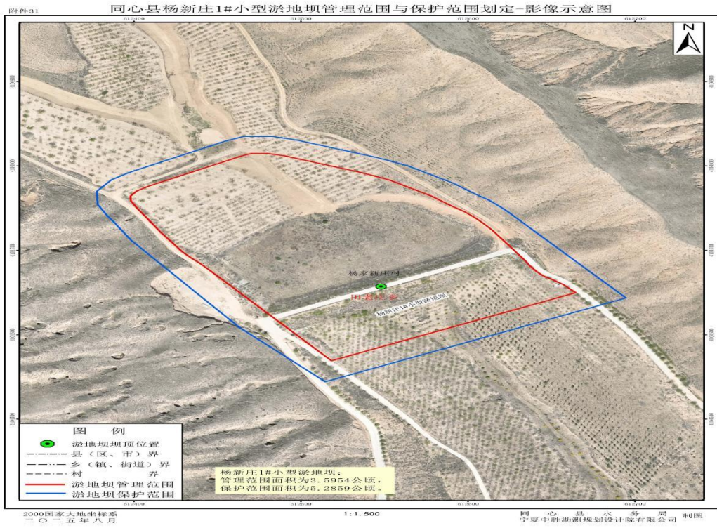
1-31 同心县杨新庄1#淤地坝管理与保护范围划定成果影像示意图
