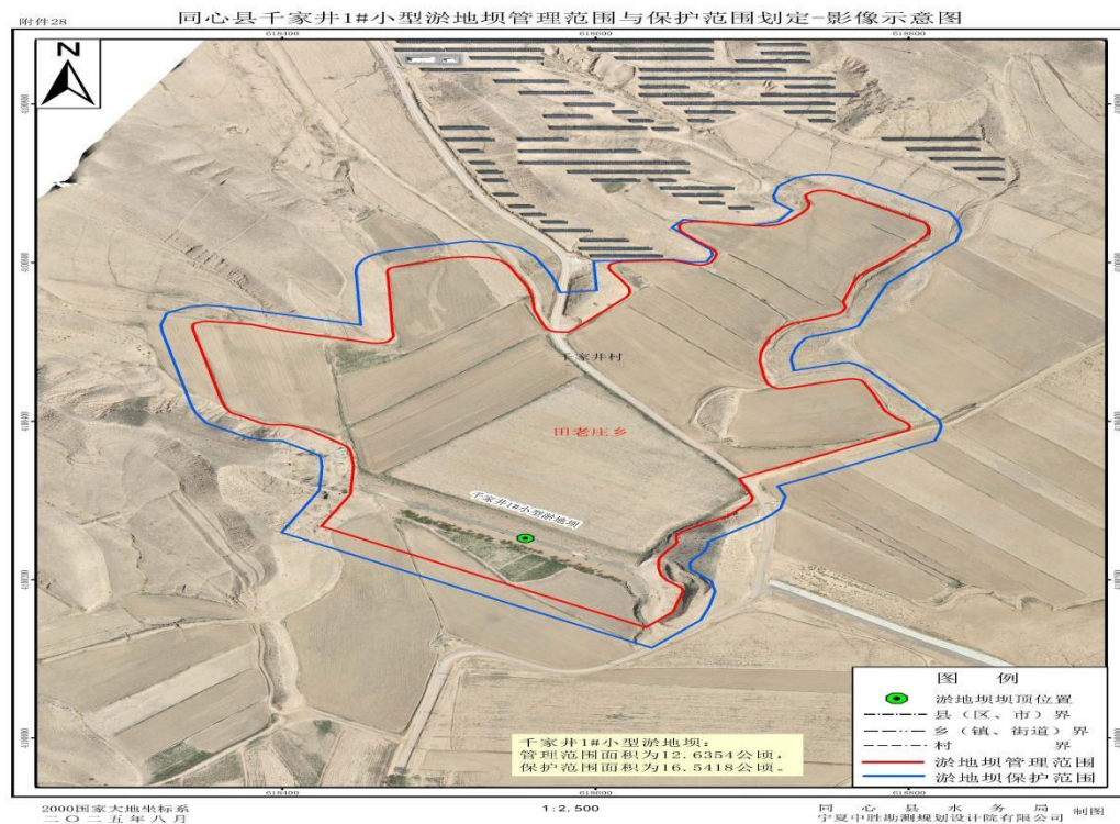
1-28 同心县千家井1#淤地坝管理与保护范围划定成果影像示意图
