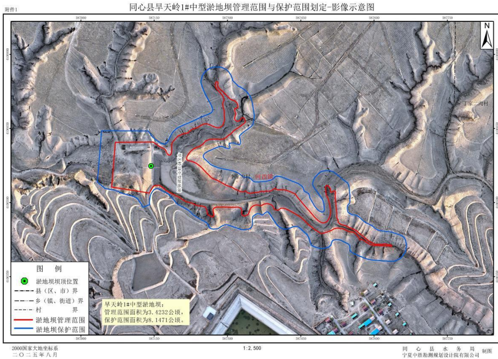
1-1 同心县早天岭1#淤地坝管理与保护范围划定成果影像示意图
