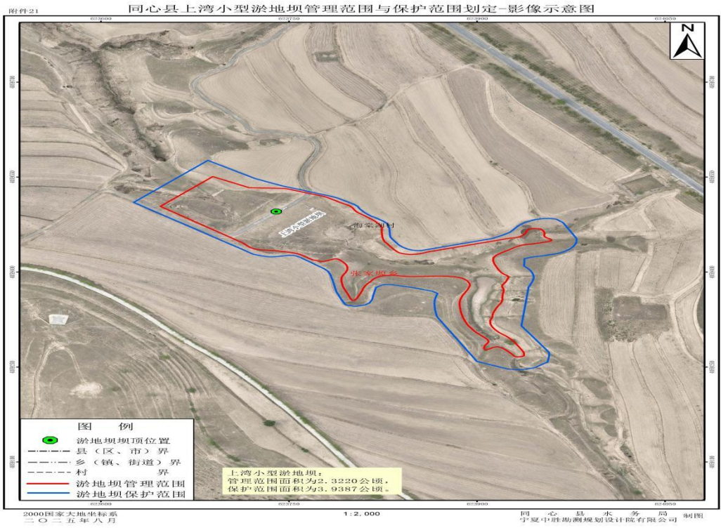
1-21 同心县上湾淤地坝管理与保护范围划定成果影像示意图
