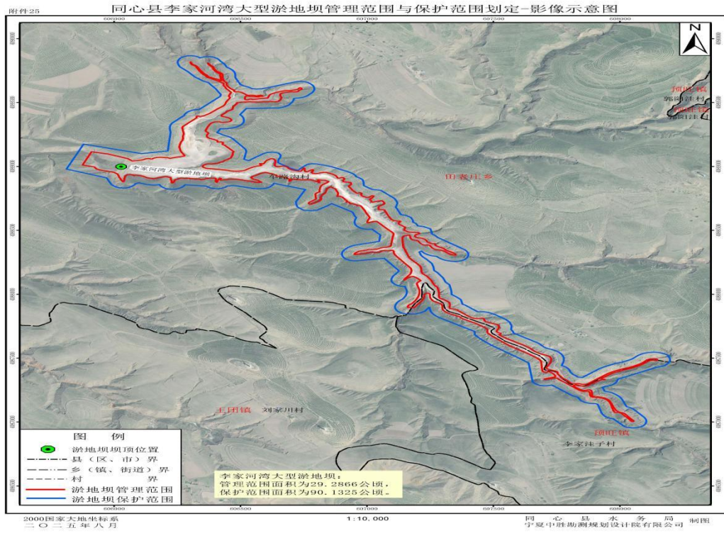
1-25 同心县李家河湾淤地坝管理与保护范围划定成果影像示意图
