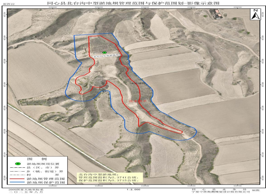
1-22 同心县北台沟淤地坝管理与保护范围划定成果影像示意图
