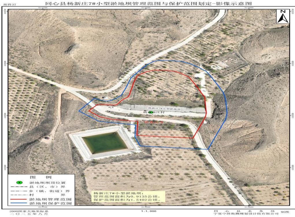
1-37 同心县杨新庄7#淤地坝管理与保护范围划定成果影像示意图
