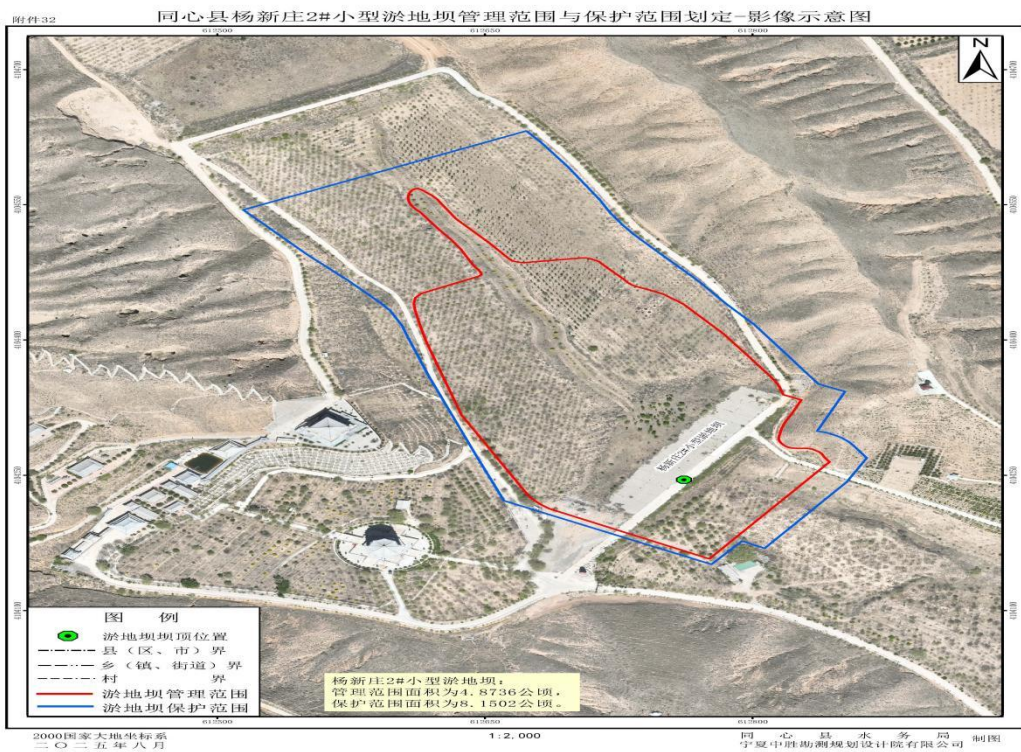
1-32 同心县杨新庄2#淤地坝管理与保护范围划定成果影像示意图
