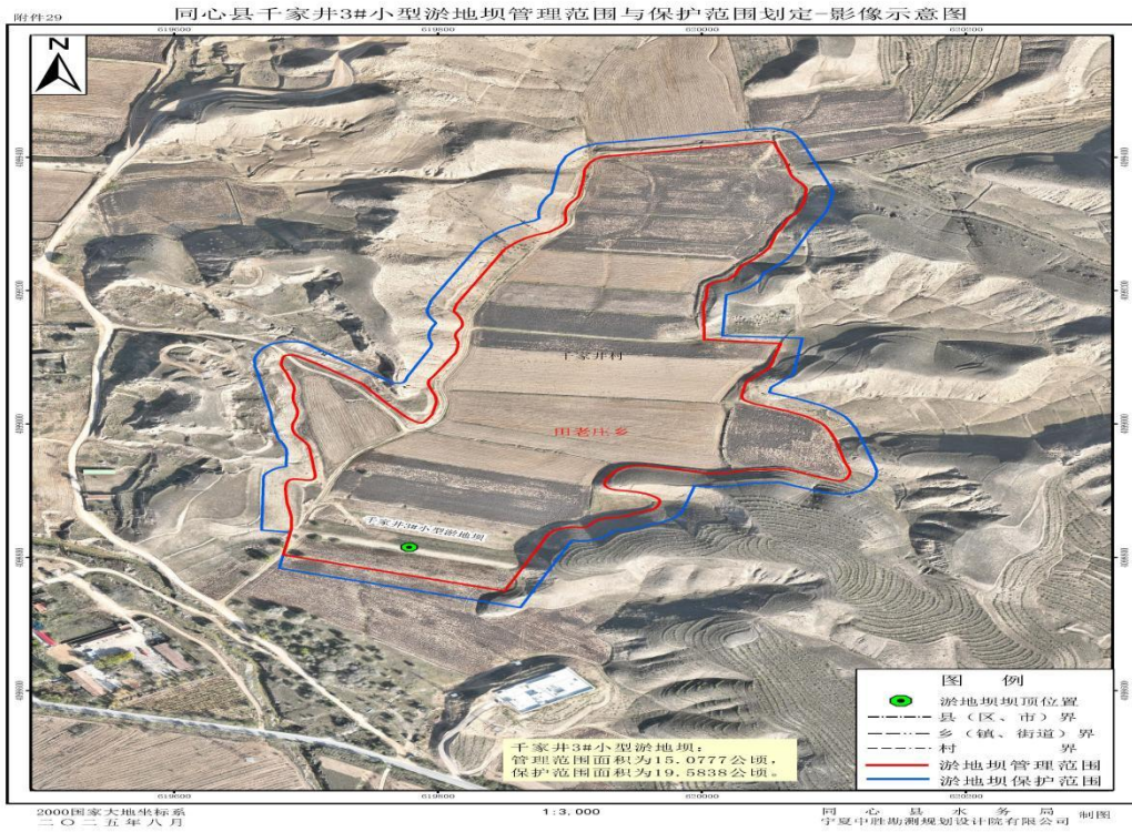
1-29 同心县千家井3#淤地坝管理与保护范围划定成果影像示意图
