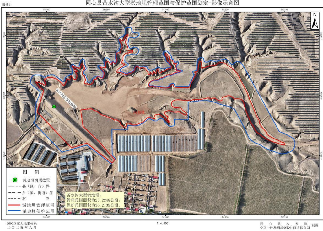
1-3 同心县苦水沟淤地坝管理与保护范围划定成果影像示意图
