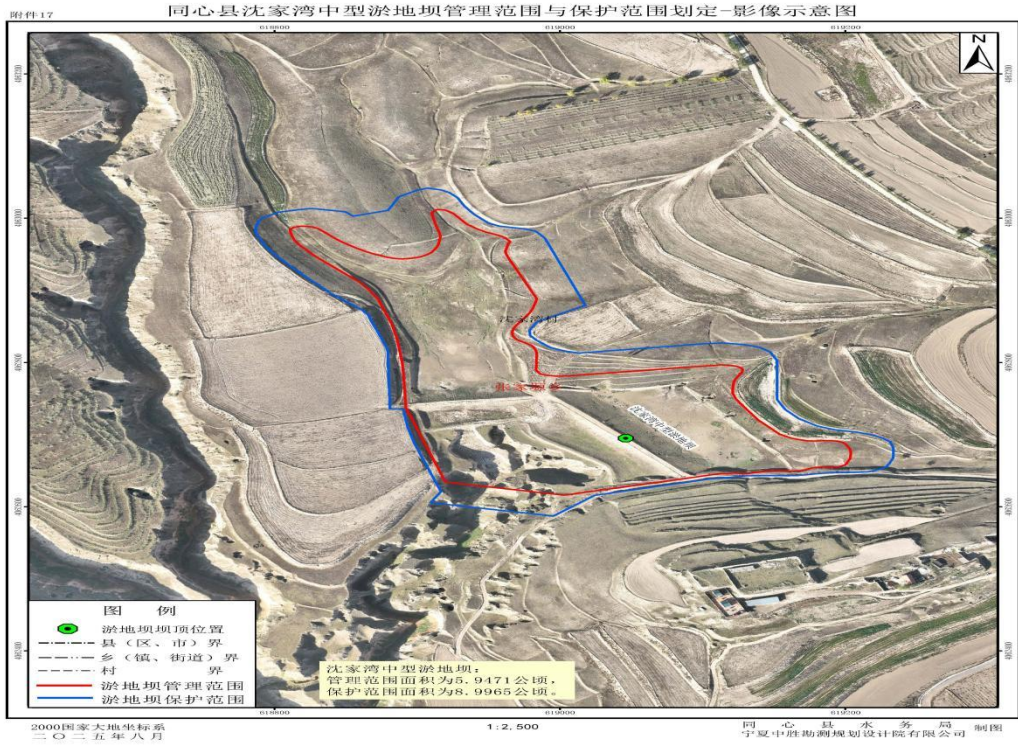
1-17 同心县沈家湾淤地坝管理与保护范围划定成果影像示意图
