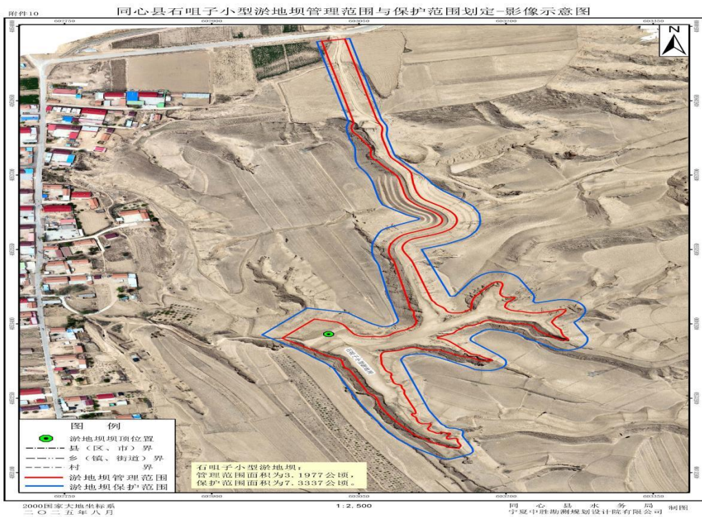
1-10 同心县石咀子淤地坝管理与保护范围划定成果影像示意图
