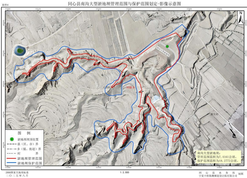
1-8 同心县南沟淤地坝管理与保护范围划定成果影像示意图
